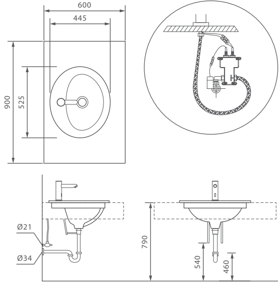
DC水龍頭標準安裝配置圖
