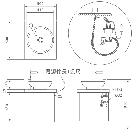
AC水龍頭標準安裝配置圖
